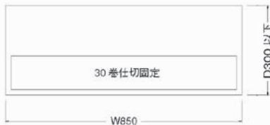
①30巻仕切固定板タイプ [収納数30巻]
